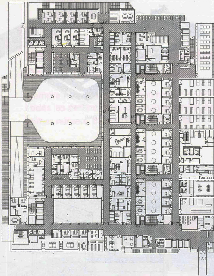
07 - PLANTA NIVEL 1 DE ACCESO DE URGENCIAS
