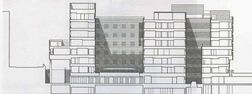
15 - SECCIÓN
