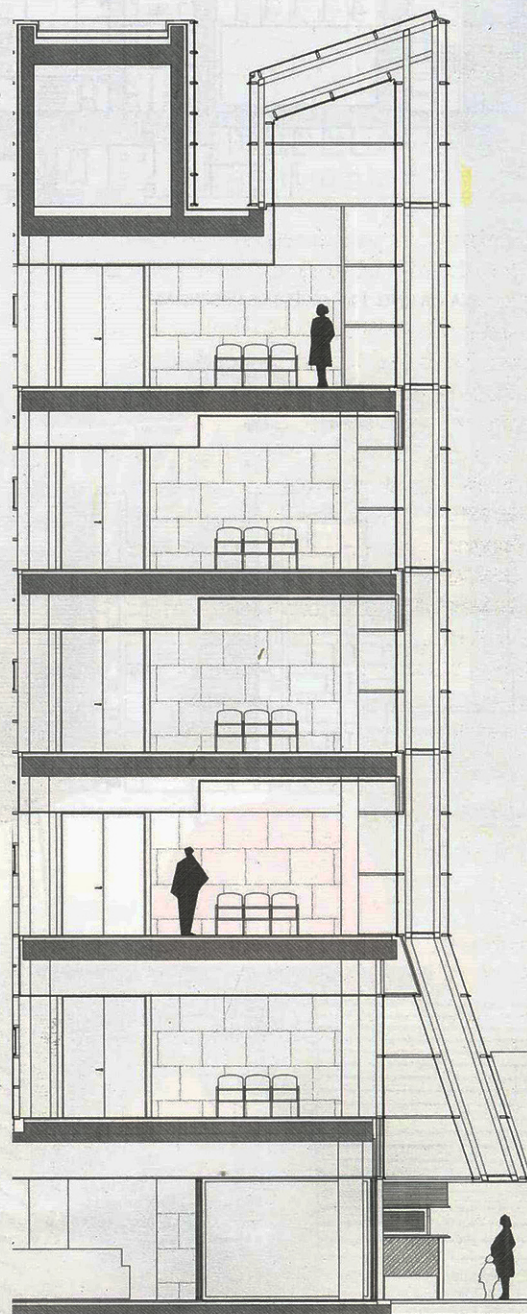
06 - DETALLE DE LA SECCIÓN POR EL VESTÍBULO DEL ACCESO A LA MATERNIDAD (O'DONELL)
