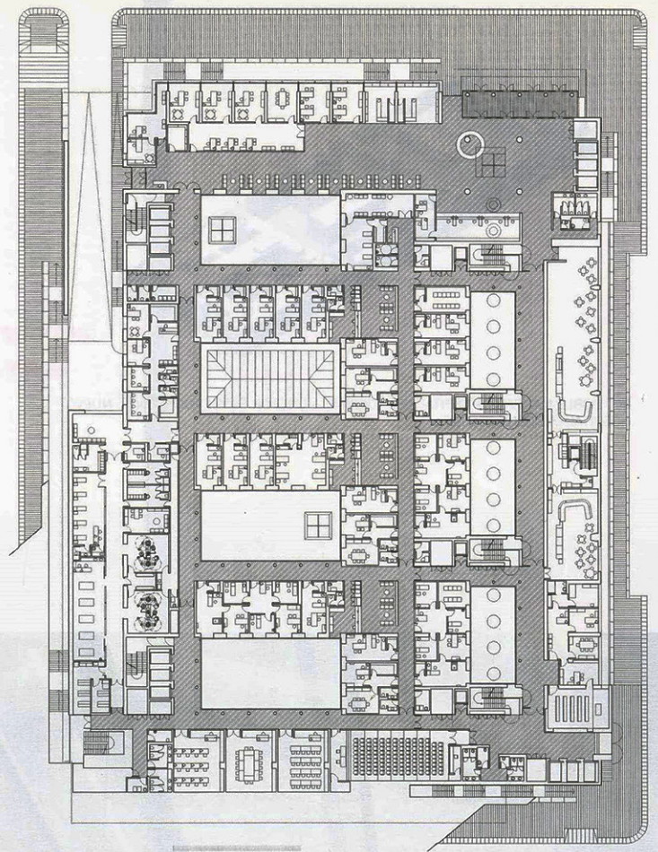
08 - PLANTA NIVEL 0 DE ACCESO DE MATERNIDAD
