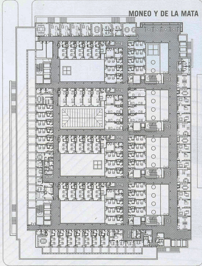
11 · PLANTA NIVEL 3 DE HOSPITALIZACIÓN PEDIÁTRICA
