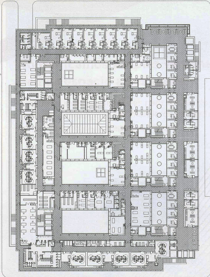
10 · PLANTA NIVEL 2 DE QUIRÓFANOS Y UVI
